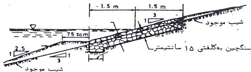
شکل (۱۱-۳) - حفاظت خاکریز اطراف دریاچه‌های تصفیه‌ی فاضلاب
